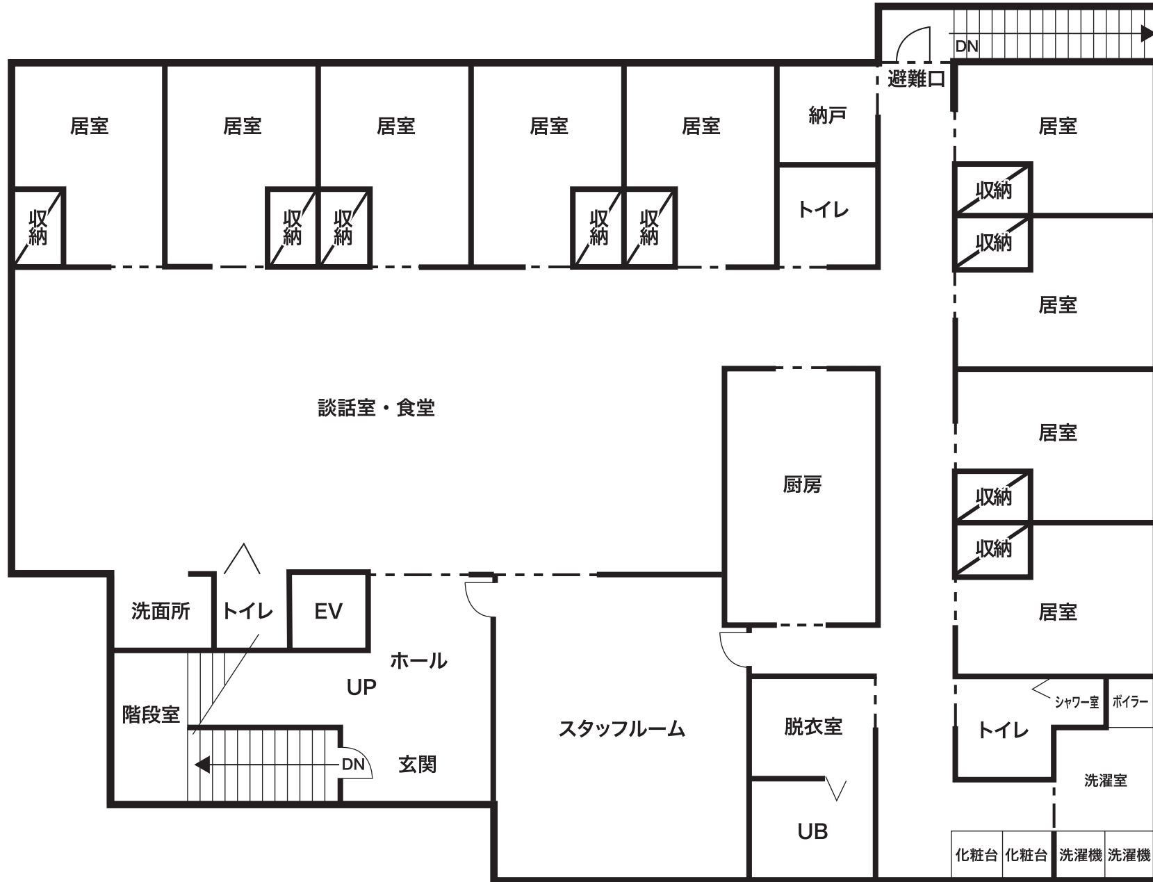
■グループホーム「ぬくもり」2F 平面図
